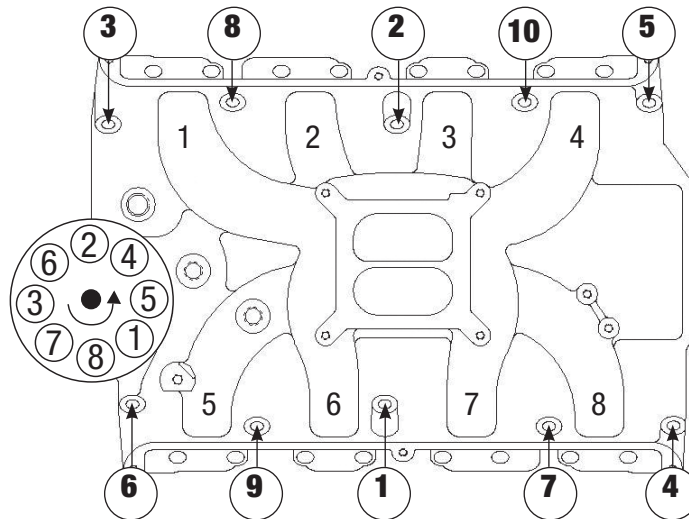
Figura 1 - 326-428 FE Ford Secuencia de Torsión Tornillos de Torsión de 25 KPa Orden de Descarga: 1-5-4-2-6-3-7-8 Gire el Distribuidor en Sentido de las Manecillas del Reloj para que Avance el Tiempo del Encendido
